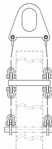
ЗКК с креплением за нижнее отверстие
