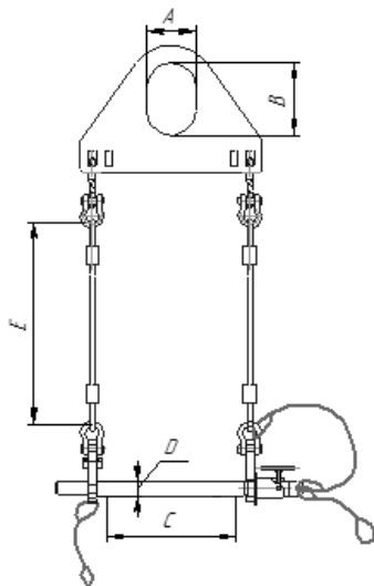
ЗКК с креплением за верхнее отверстие
